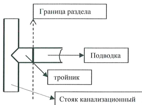
Рис. 1. Сети водоотведения (канализация)
